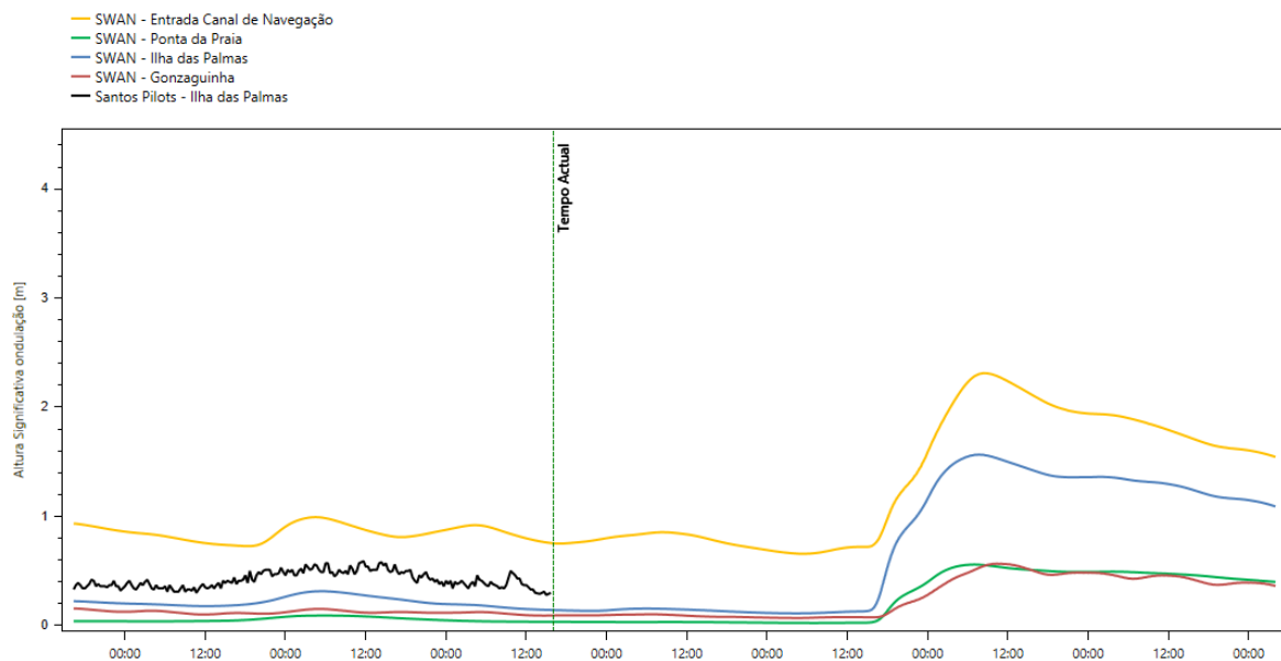
Figura 2. Previsão do modelo de ondas. A altura significativa da onda (m) para as regiões da entrada do canal de navegação (linha em laranja), Ilha das Palmas (linha azul), Ponta da Praia (linha verde) e Gonzaguinha (linha vermelha), dados coletados pelo sensor da Praticagem de Santos em preto.
