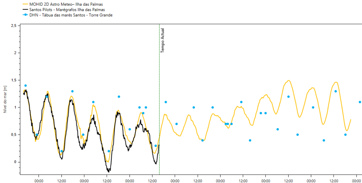
Figura 1. Previsão do modelo hidrodinâmico (linha laranja), apresentando o nível do mar (maré) na estação da Ilha das Palmas. A previsão da Tábua de Marés está representada em azul e os dados coletados pelo marégrafo da Praticagem de Santos estão apresentados em preto.
